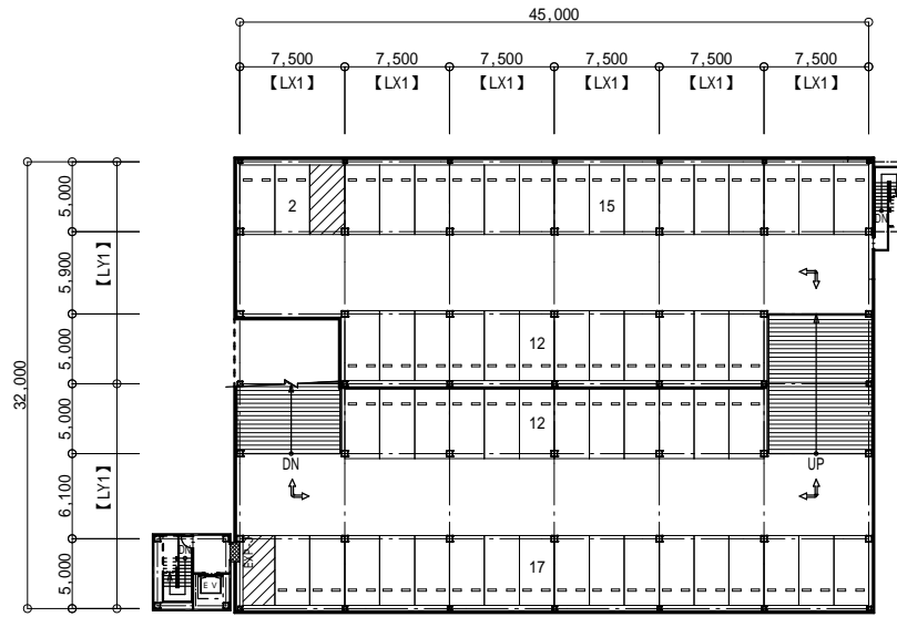
R階 平面図
