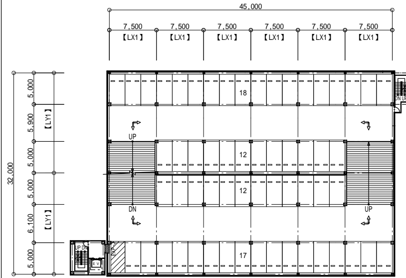
2 ~ 6階 平面図
