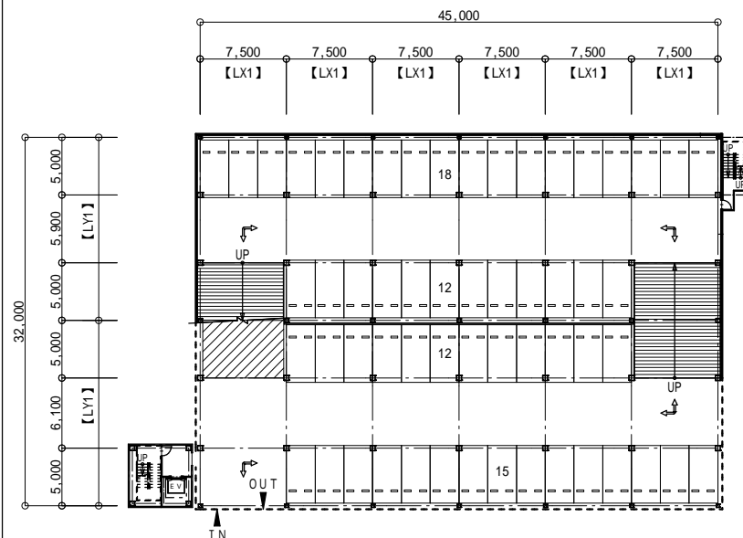
1階 平面図
